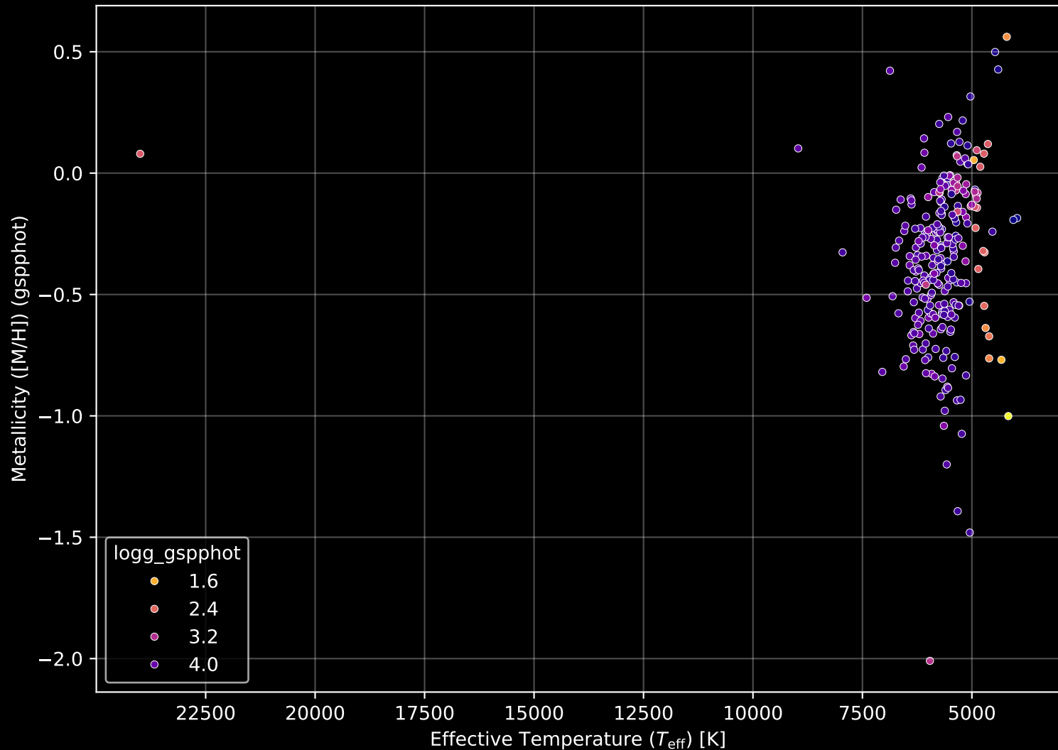
GALAH DR4 Field: [1145] Stellar Population Parameters (n= 269)
