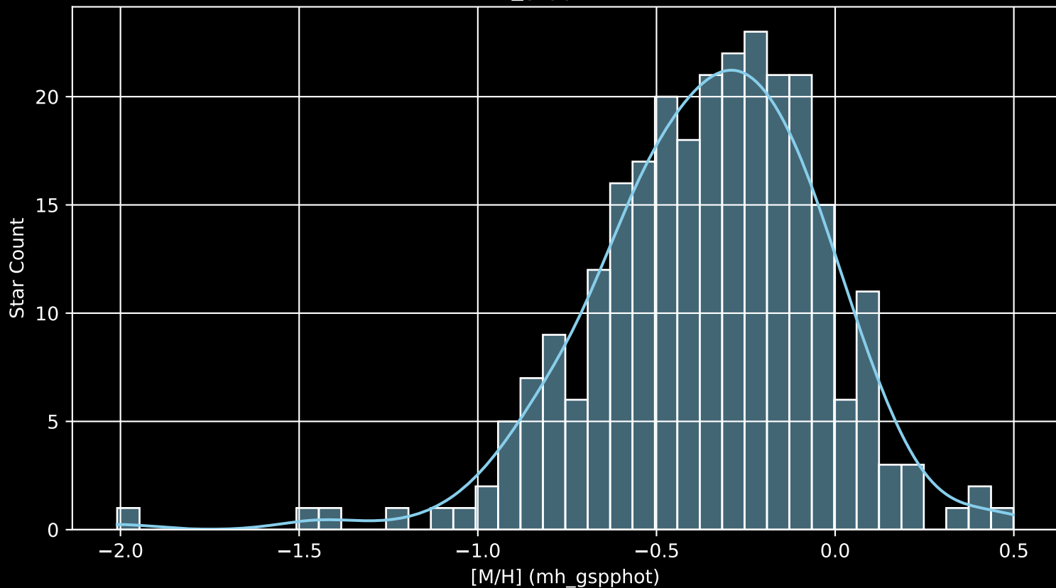
GALAH DR4 Field: [1145] [M/H] (mh_gspphot) (n= 268)
