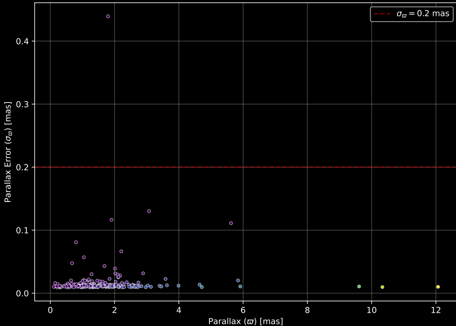
GALAH DR4 Field: [1145] Parallax Quality (n= 269)
