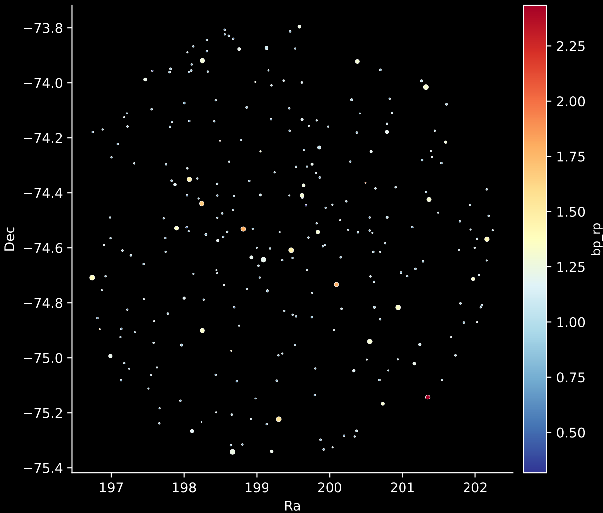
GALAH DR4 Field: [1145] Stars: 269
